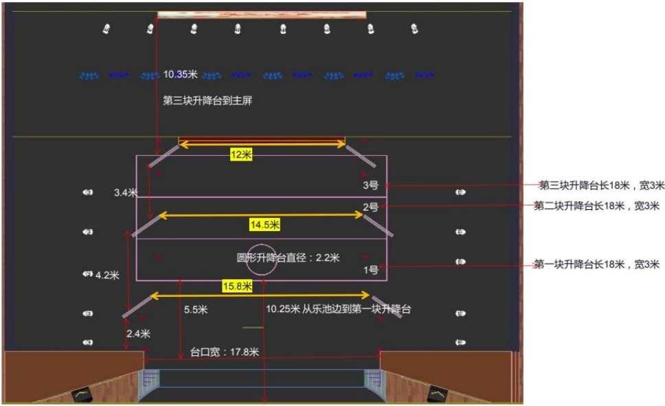
璧山文化艺术中心平面图
