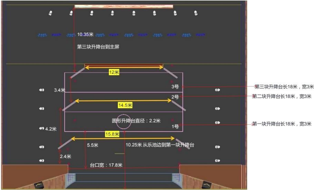
璧山文化艺术中心平面图
